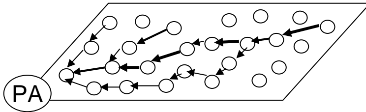
RSSF plana
