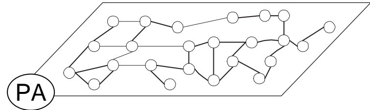
Auto-organização
