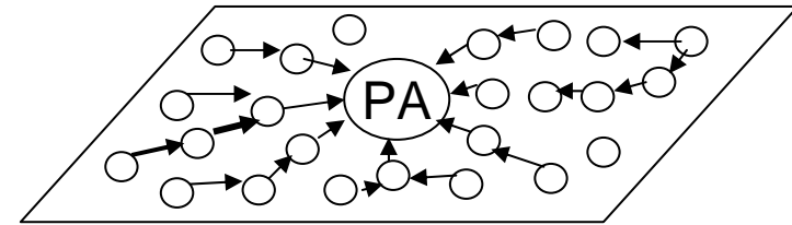
RSSF plana
