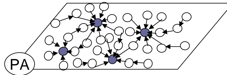
RSSF hierárquica
