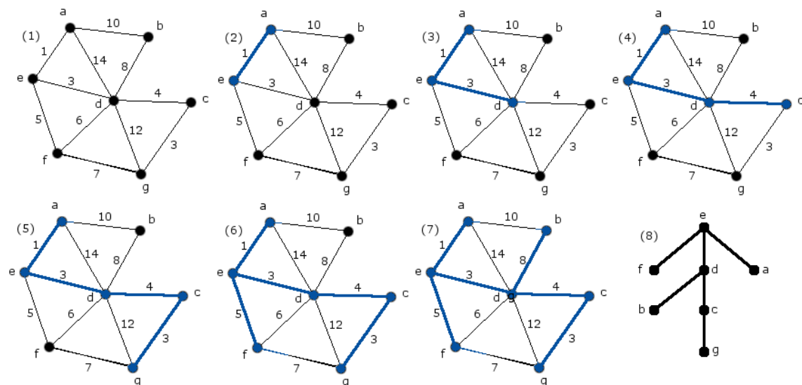
Figura 15 - Sequência de formação da árvore geradora mínima a partir de um grafo utilizando o algoritmo de Prim.
