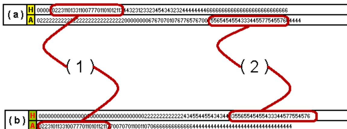
Figura 9 - Região de combinação entre os códigos de cadeia de Freeman entre as partes: (1), parte (a) sentido horário e (b) anti-horário; (2), parte (a) sentido anti-horário e (b) horário.
