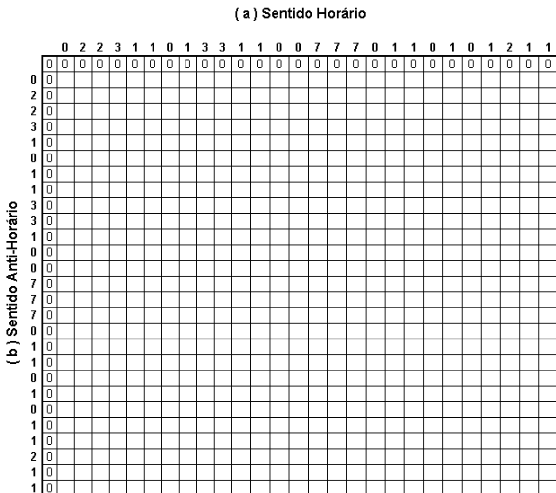
Figura 10 - Matriz inicial para o algoritmo de LCS: (a) Parte da sequência no sentido horário; (b) Parte da sequência no sentido anti-horário.
