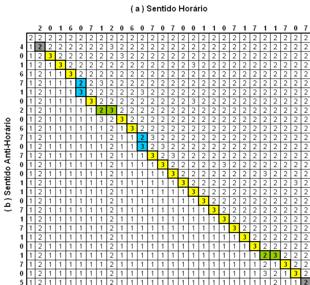
Figura 46 - Matriz backtracking para as cadeias de complemento.
