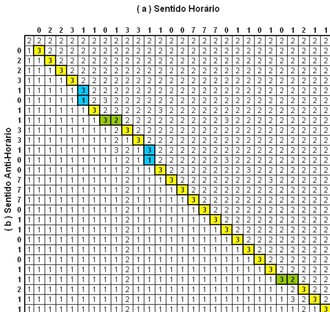
Figura 12 - Matriz de backtracking calculada para as subsequências de cadeias de códigos de Freeman.
