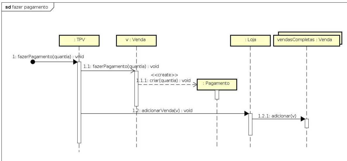
Figura 5: Diagrama de sequência para a operação Fazer Pagamento
