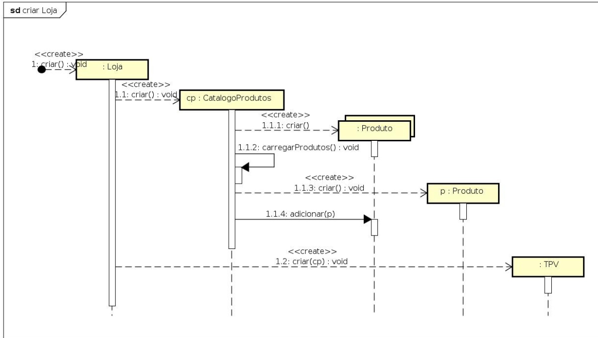
Figura 2: Diagrama de sequência para a operação Criar Loja
