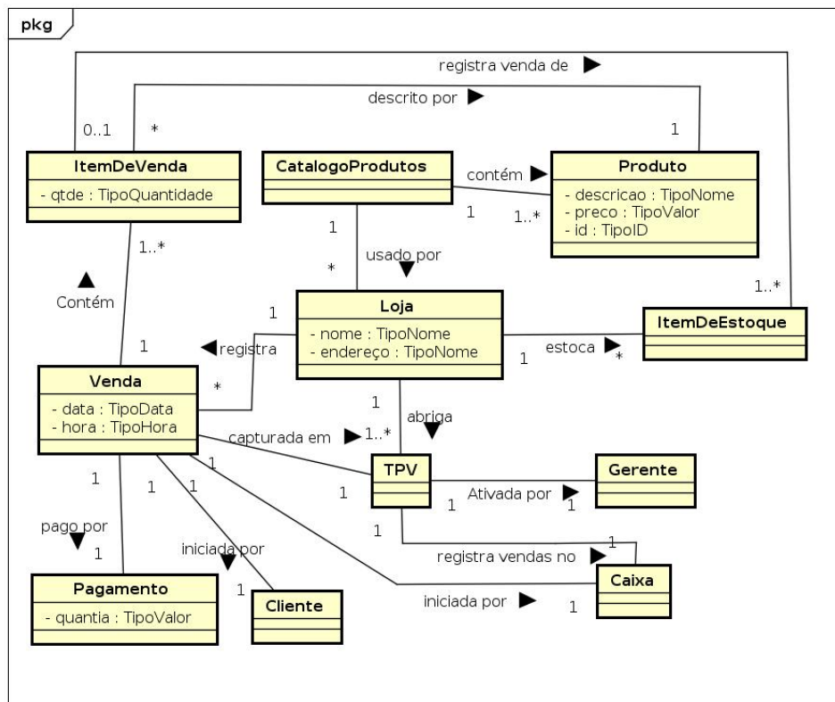
Figura 1: Diagrama de classes conceituais para o Sistema de Ponto de Vendas
