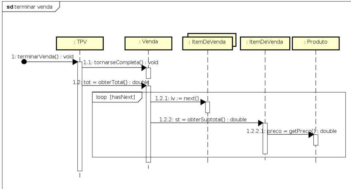
Figura 4: Diagrama de sequência para a operação terminar Venda
