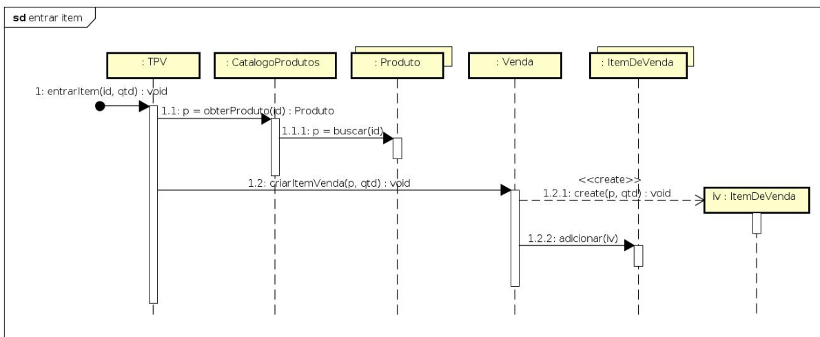
Figura 3: Diagrama de sequência para a operação Entar Item
