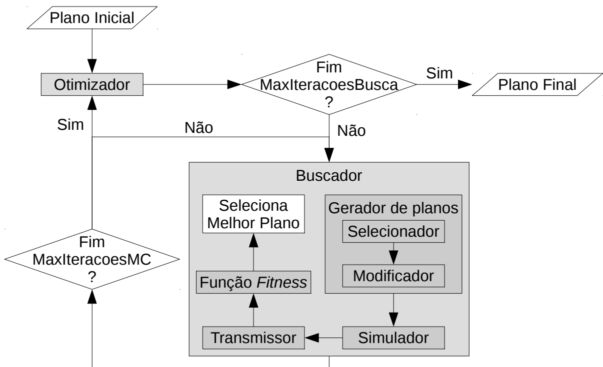
Figura 4.1: Fluxograma da solução proposta
