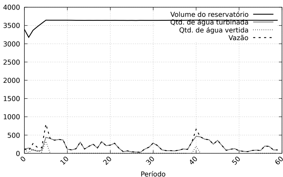
Figura 4.4: Resultados da simulação com um plano conservador
