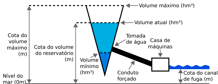
Figura 1.3: Componentes de uma usina hidrelétrica com reservatório
