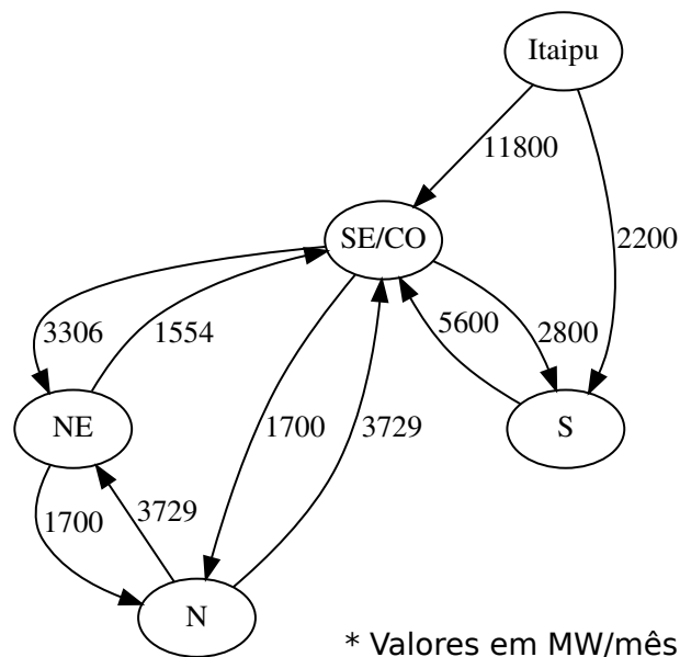
Figura 2.3: Grafo de transmissao
