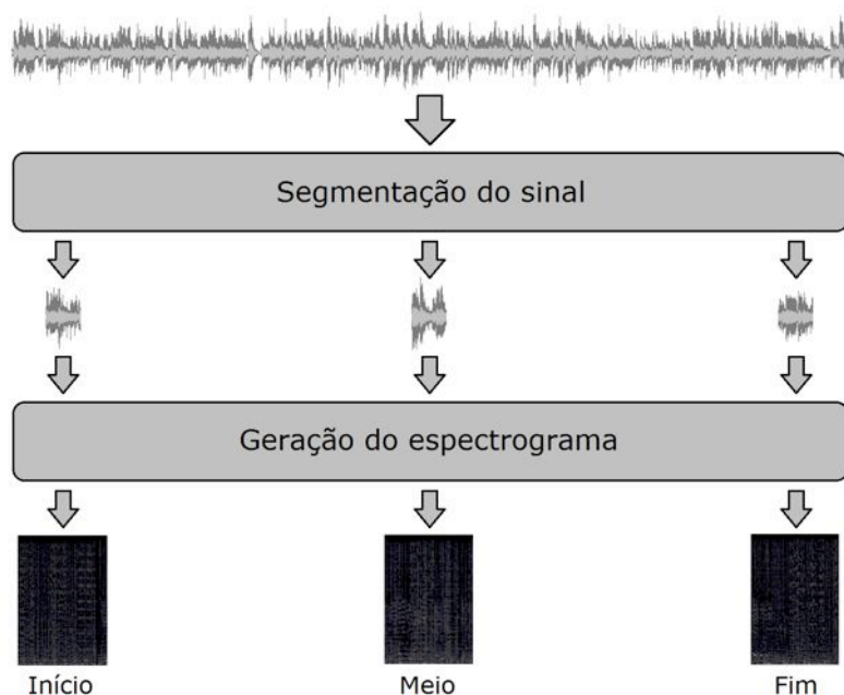
Figura 4.2: Segmentação do sinal e geração dos espectrogramas.
