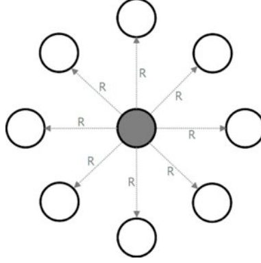
Figura 3.9: Operador LBP. Pixel C , círculo escuro ao centro, seus P vizinhos, círculos claros.
