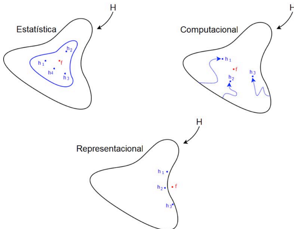
Figura 3.11: As três diferentes razões para combinar classificadores [15].
