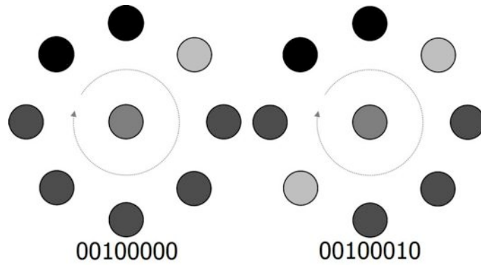
Figura 3.10: Uniformidade do padrão LBP. (a) com apenas duas transições, o padrão é considerado uniforme. (b) com quatro transições, o padrão não é considerado uniforme.
