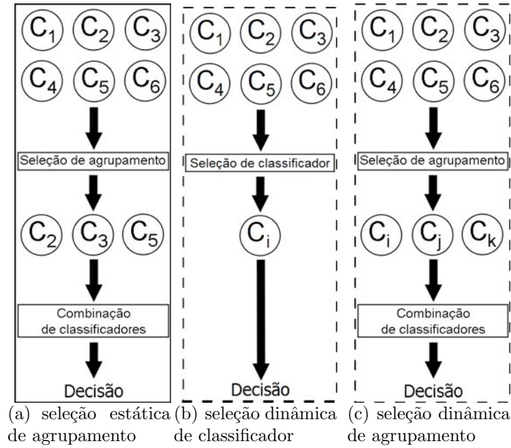
Figura 3.13: Esquemas utilizados na seleção de classificadores [43].
