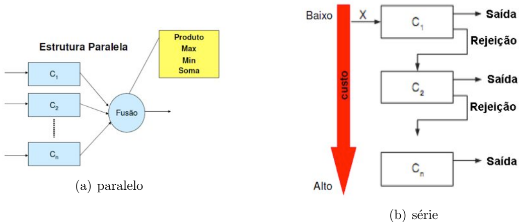
Figura 3.12: Arquiteturas para combinação de múltiplos classificadores.
