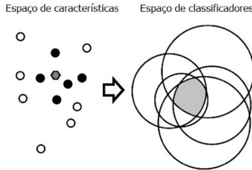
Figura 3.14: KNORA ELIMINATE utiliza apenas os classificadores que classificam corretamente todos os K padrões mais próximos. O hexágono corresponde ao padrão de teste, os padrões do conjunto de validação são os circulares, sendo que os 5 mais próximos estão em preto [43].
