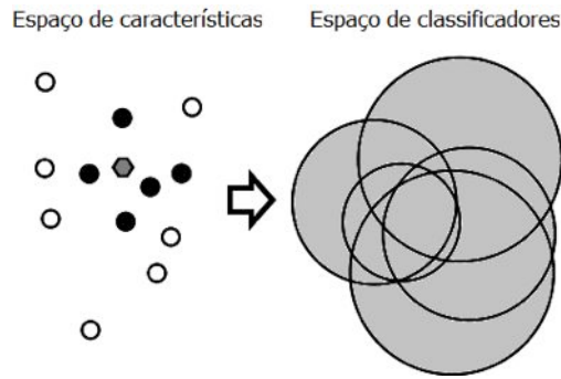
Figura 3.15: KNORA UNION utiliza os classificadores que classificam corretamente algum dos K padrões mais próximos. O hexágono corresponde ao padrão de teste, os padrões do conjunto de validação são os circulares, sendo que os 5 mais próximos estão em preto [43].
