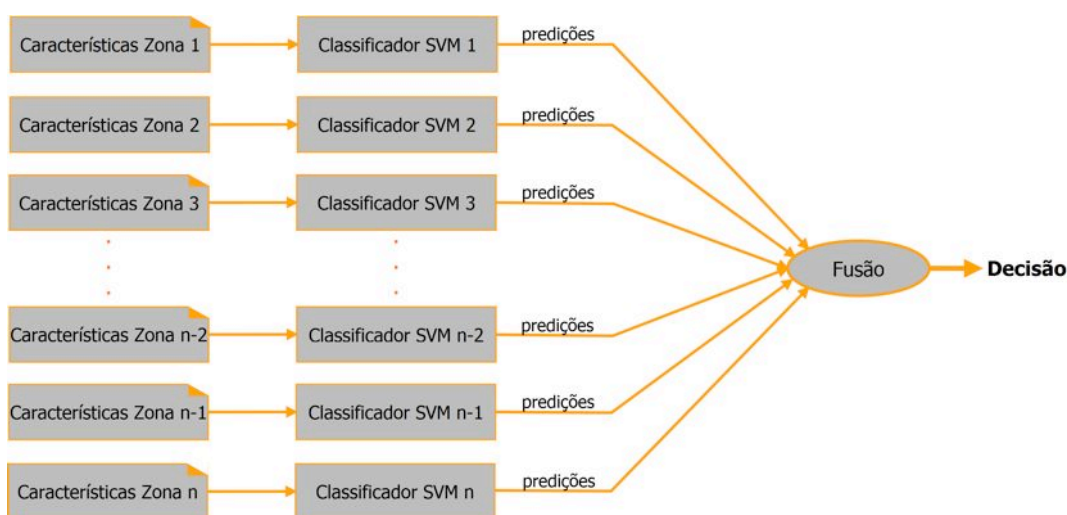
Figura 4.4: Criação de classificadores para as características extraídas de cada zona e fusão das saídas.
