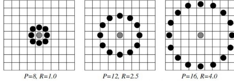
Figura 4.11: Exemplos de possíveis vizinhanças utilizadas em LBP [61]
