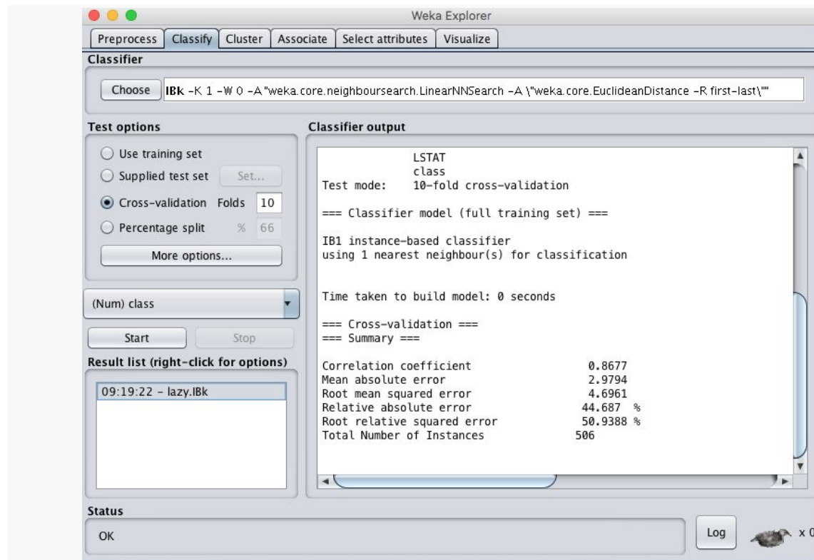
Resultados da Regressão Weka para o Algoritmo k-Nearest Neighbours
