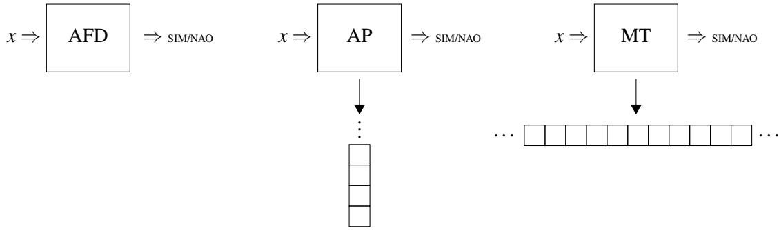
Figure 5.1: Comparação entre um AFD, um AP e uma Máquina de Turing. Os AFDs são máquinas de estados e APs são máquinas de estados com acesso a uma memória em forma de pilha de dados. A Máquina de Turing é essencialmente uma máquina de estados com uma memória em forma de fita de dados. A máquina pode acessar diferentes posições desta fita e ler/escrever um símbolos em tais posições.
