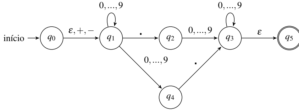
Figure 3.5: Um \varepsilon -AFN que aceita números decimais.
