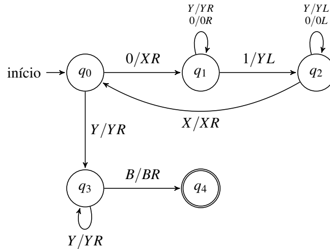
Figure 5.4: Diagrama de estados de uma Máquina de Turing.
