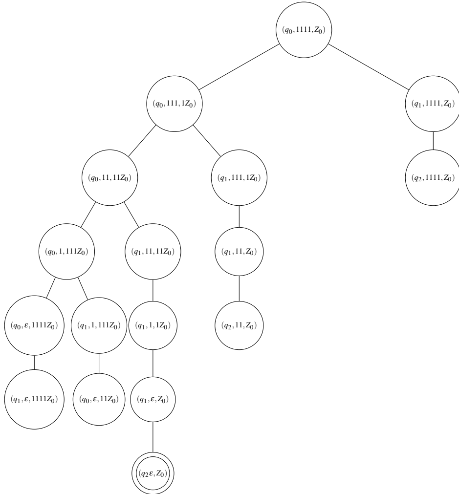
Figure 4.3: A árvore de computações possíveis do AP P_{RR} da Figura 4.2 com a string 1111. O nó marcado com dois círculos concêntricos é um nó que corresponde a uma configuração em que o AP aceita a string de entrada.
