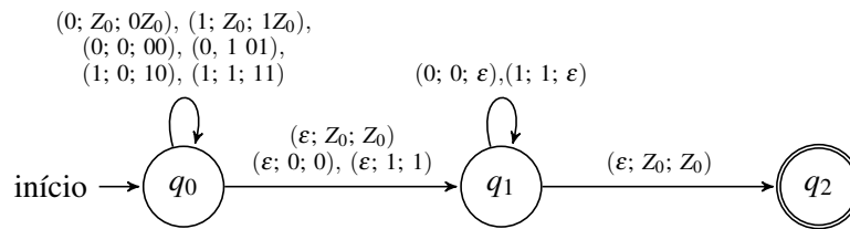
Figure 4.2: Diagrama do autômato com pilha para a linguagem dos palíndromos de tamanho par.
