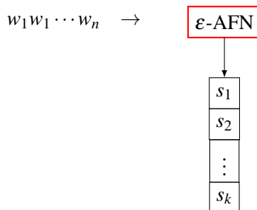
Figure 4.1: Esquema conceitual de autômatos com pilha.
