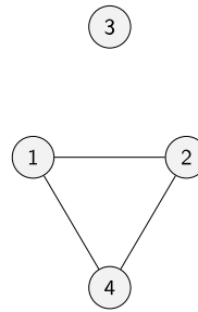
um grafo desconexo
