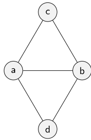
um grafo conexo
