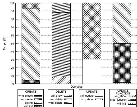
Figura 4. Tempo de execução das suboperações em porcentagem.
