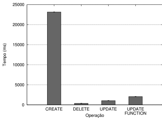
Figura 3. Tempo total de execução das operações.
