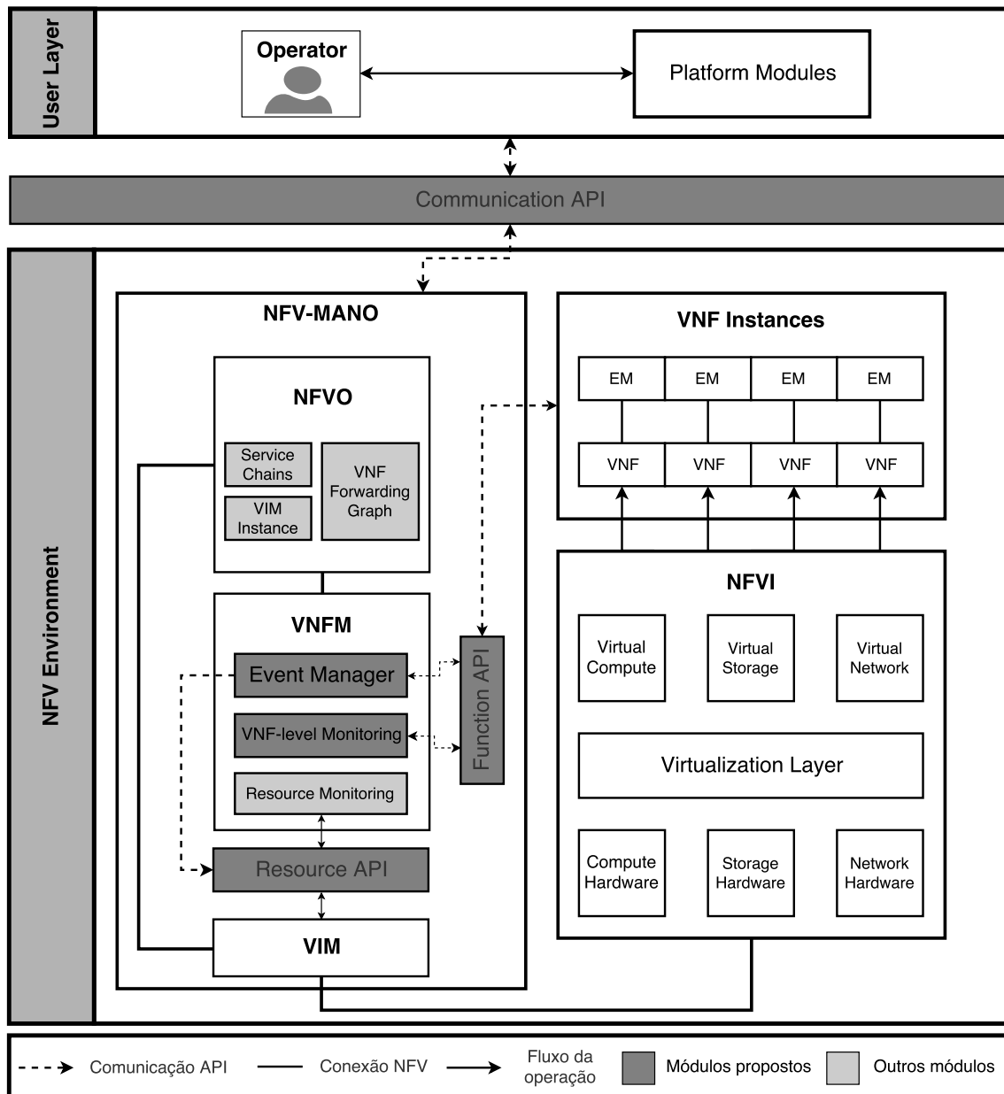
Figura 2. Arquitetura onde o VNFM está inserido.
