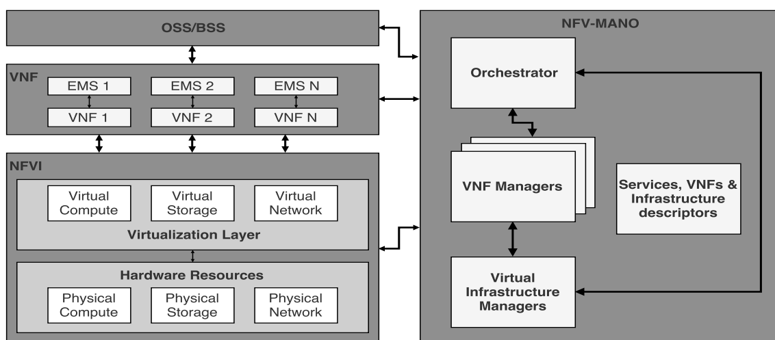
Figura 1. Arquitetura NFV.
